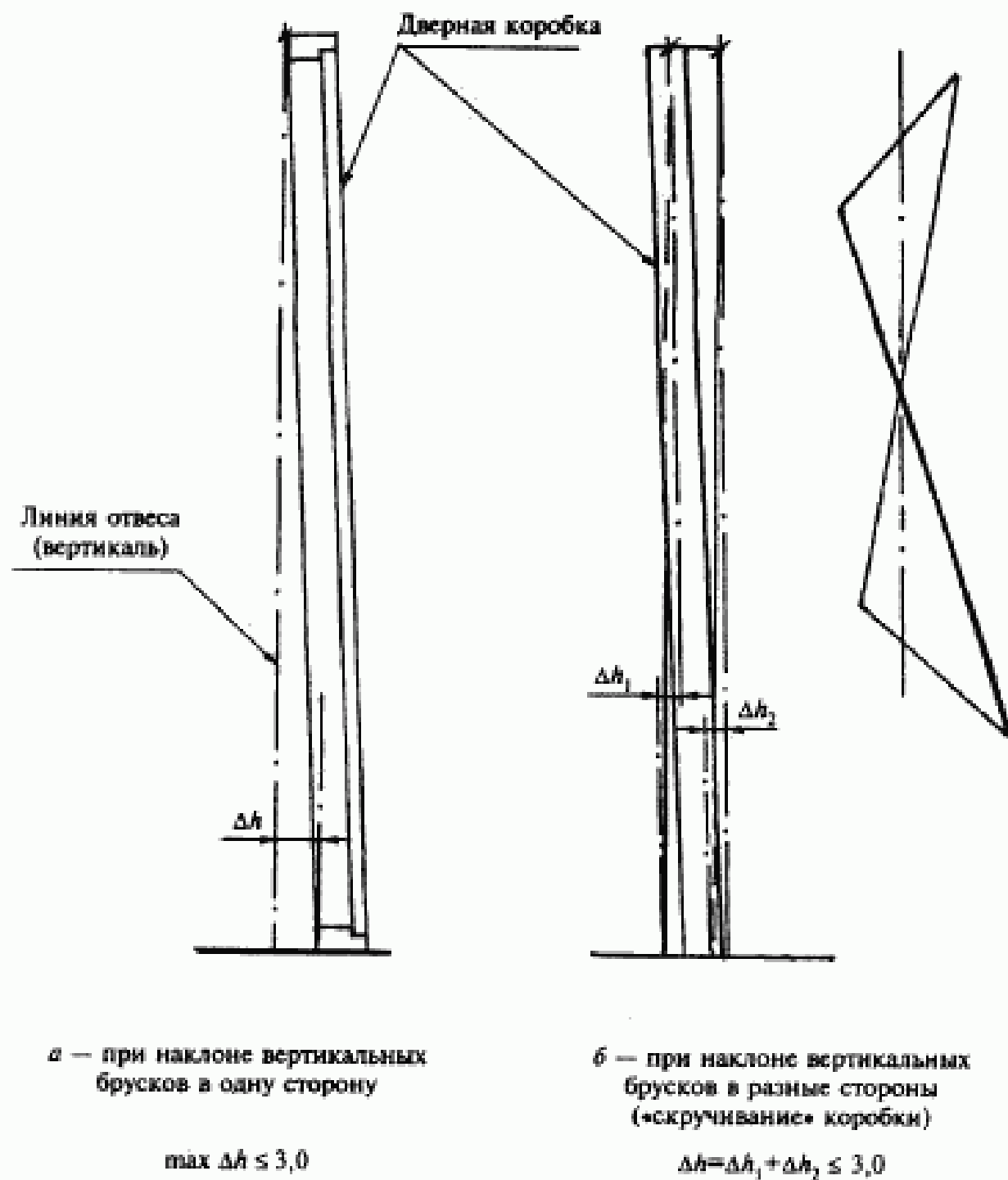
Рисунок В.2 — Определение отклонений дверной коробки
