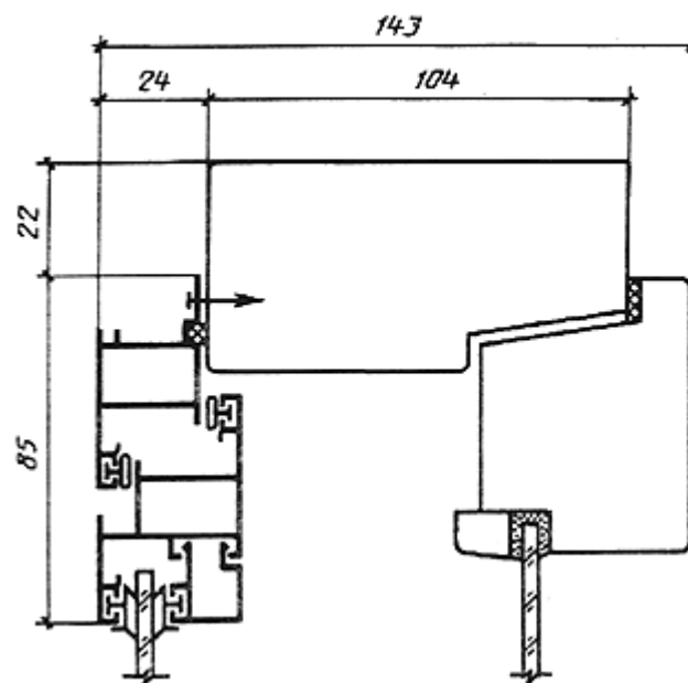
Черт.2 Сечение 2
