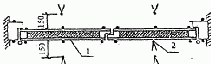
Рисунок 3 — Схема размещения термопар и термометров на образце дверного блока
